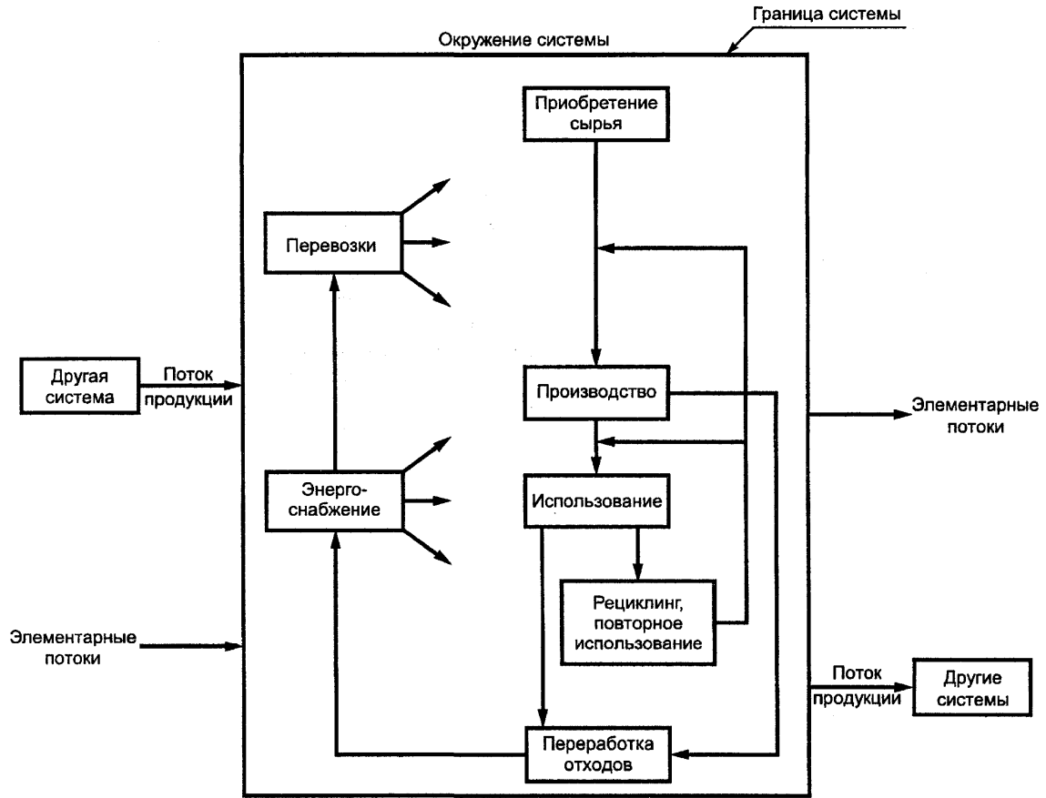
Рисунок 1 — Пример производственной системы
